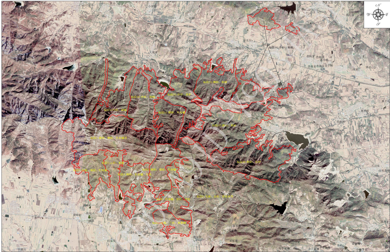
伟德山生态修复工程标段划分示意图 1:20,000
