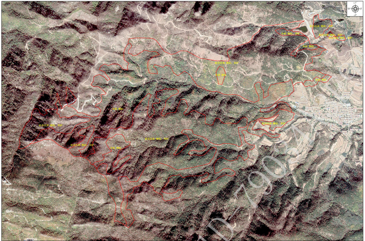
荣成市伟德山生态修复工程造林项目标段十五设计图 1:8,000
