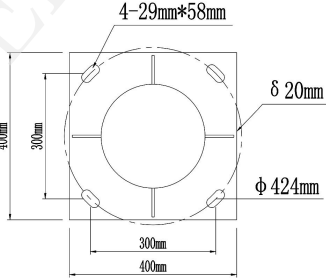
路灯底座法兰盘
