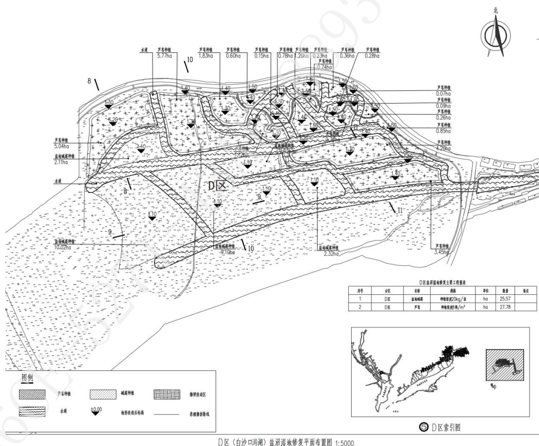
图 1.3-3 白沙口瀉湖盐沼湿地修复平面布置图
