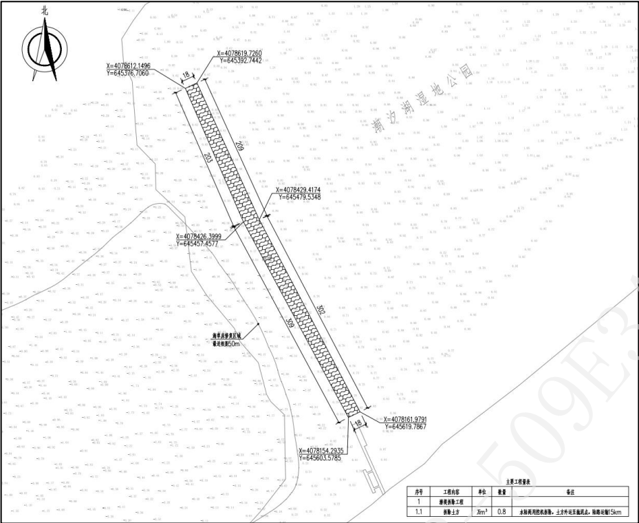
图 1.3-5 潟湖中部潜堤拆除平面布置图
