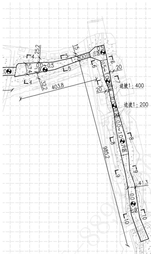
图 1.4-1 白沙滩河河道疏通底标高
