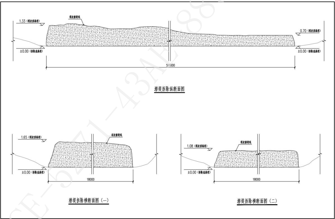
图 1.3-6 潟湖中部潜堤拆除断面图图
