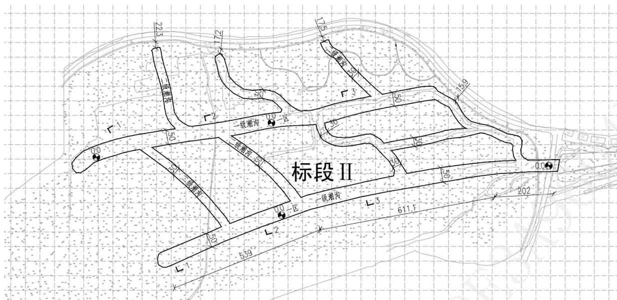
图 1.3-2 白沙滩河河道疏通底标高
