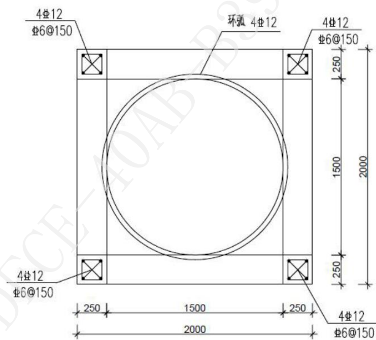
B-B 断面配筋图
