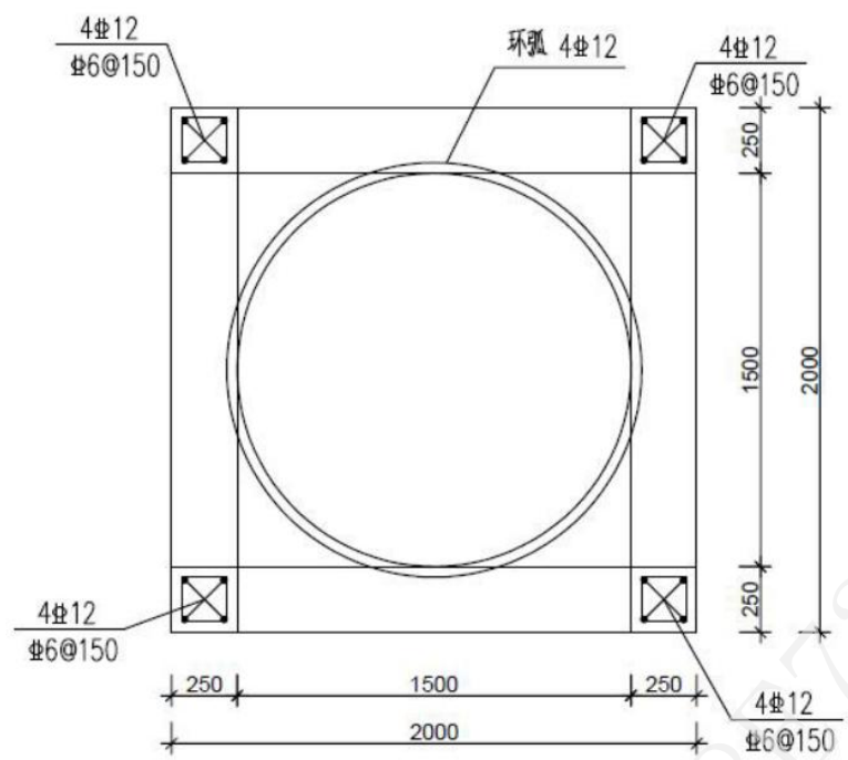
A-A 断面配筋图
