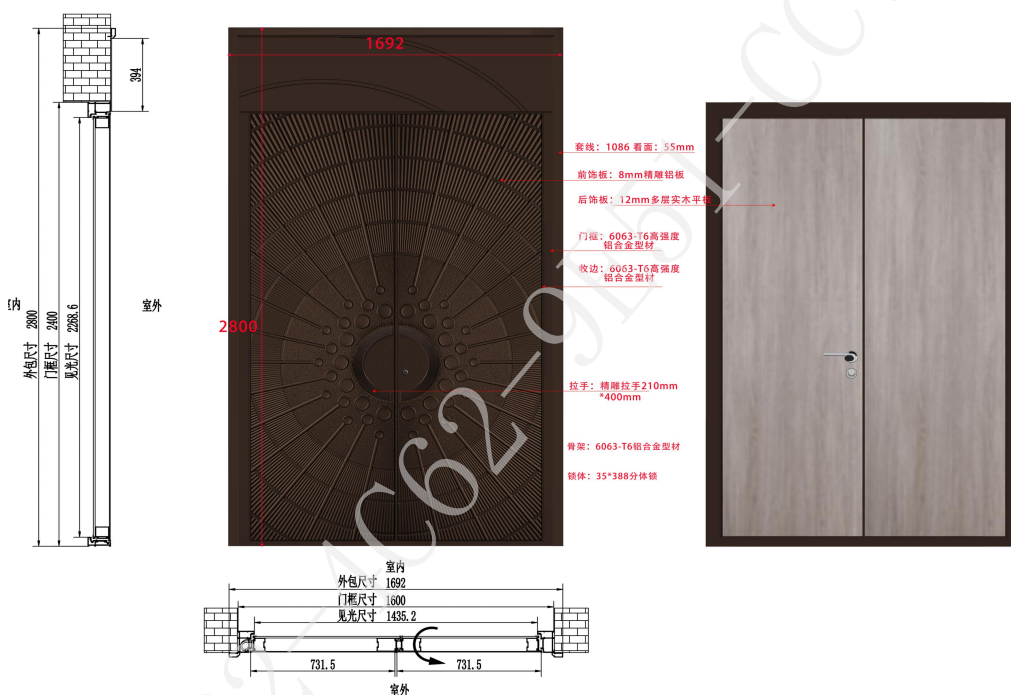
铸铝门门样图（1）单门、子母门、双开门
